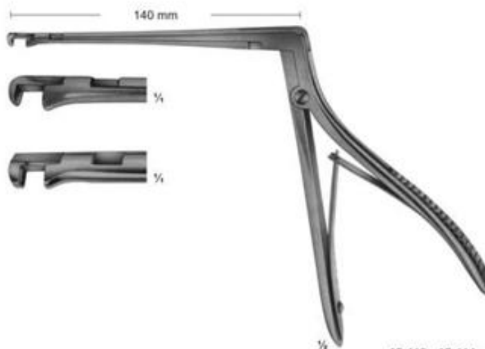
15-113 - 15-114 HAJEK-KOFLER
