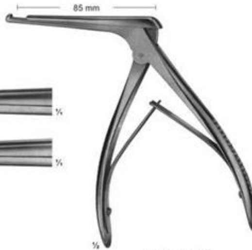
15-111 - 15-112 KERRISON
